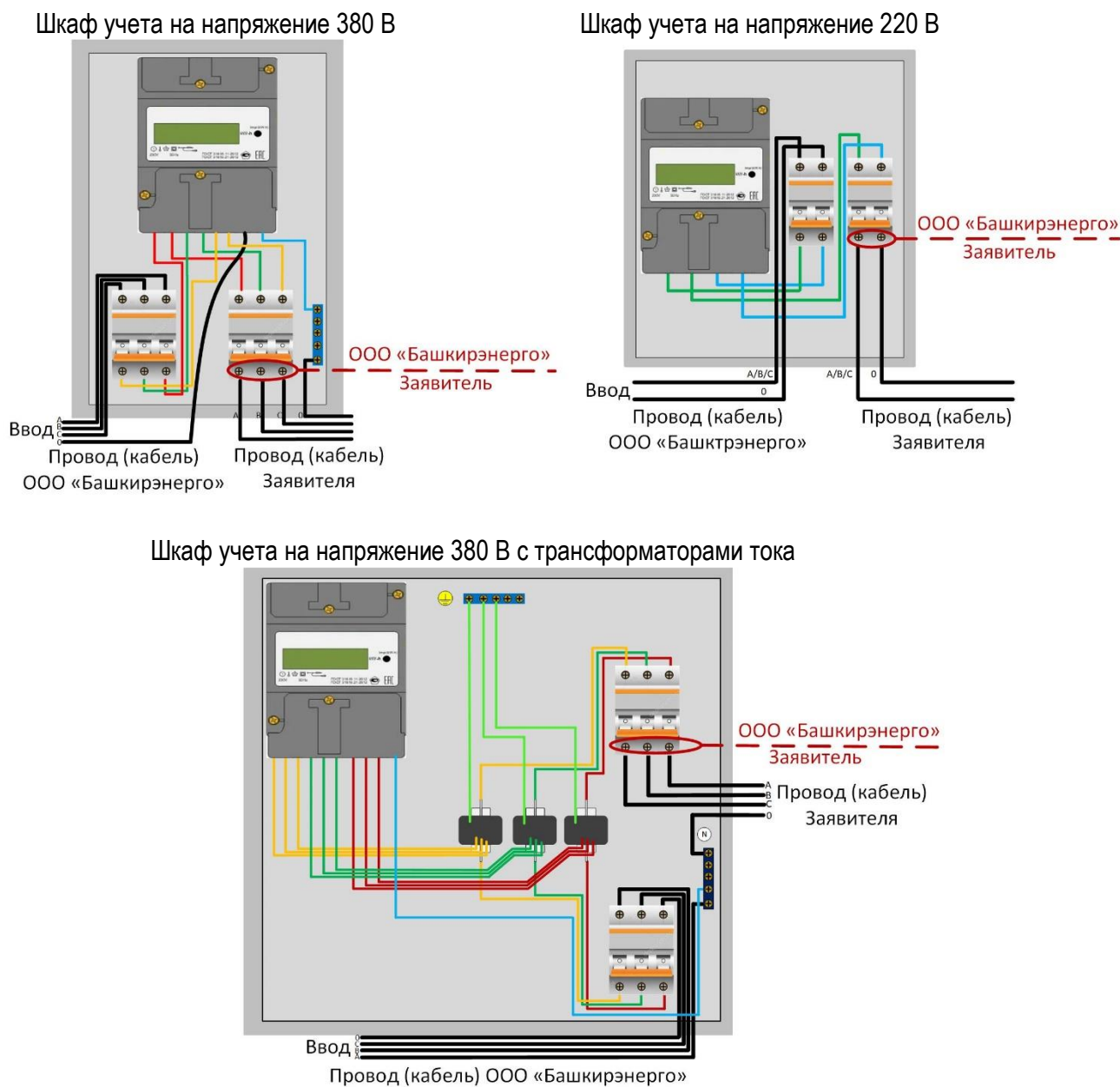
Рис. 4. Схема присоединения электрических контактов с указанием границ балансовой принадлежности сторон в шкафу учета.
