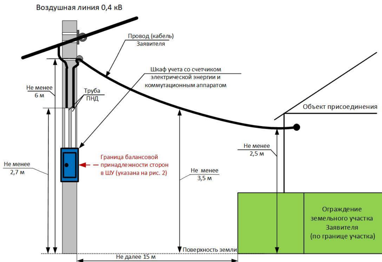
Рис. 1. Схема присоединения объекта Заявителя к электрическим сетям ООО «Башкирэнерго».
