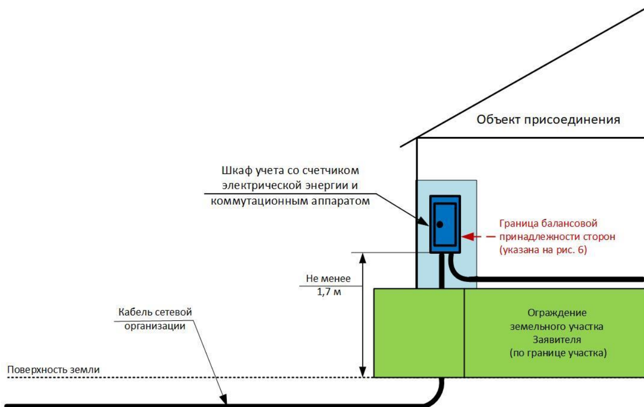
Рис. 5. Схема присоединения объекта Заявителя к электрическим сетям ООО «Башкирэнерго».
