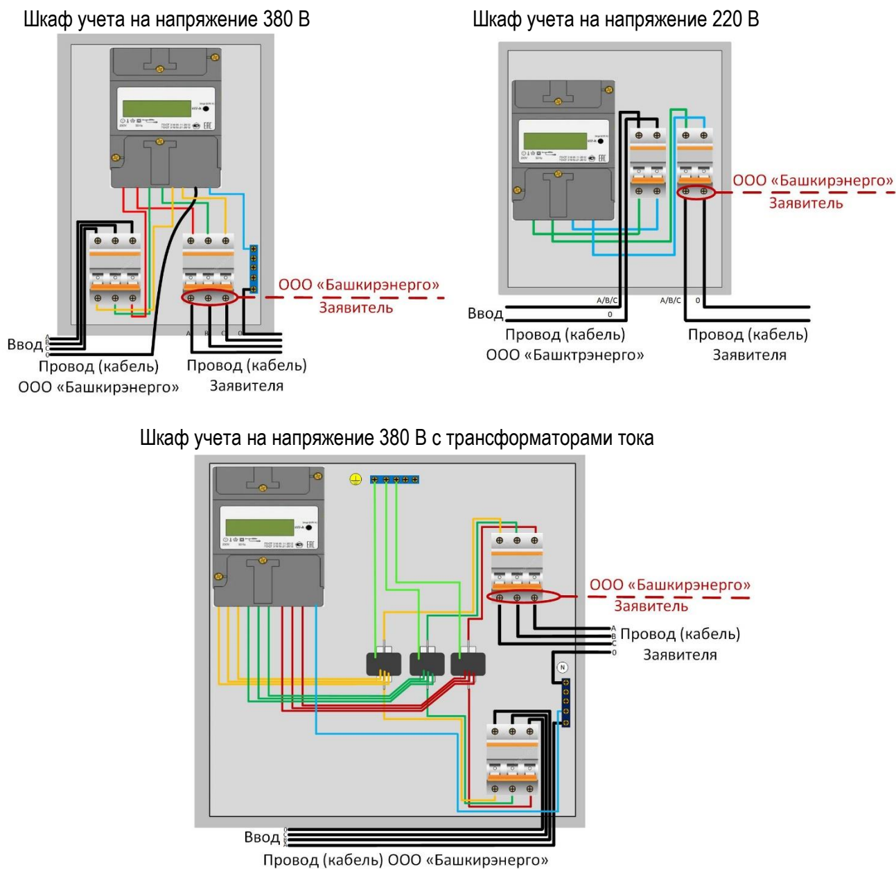
Рис. 6. Схема присоединения электрических контактов с указанием границ балансовой принадлежности сторон в шкафу учета.
