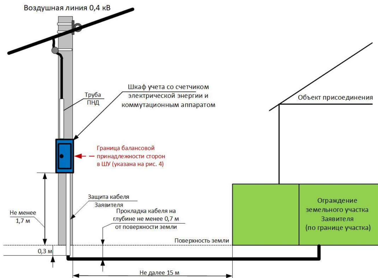
Рис. 3. Схема присоединения объекта Заявителя к электрическим сетям ООО «Башкирэнерго».
