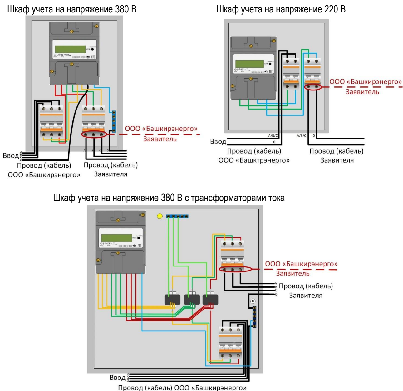
Рис. 2. Схема присоединения электрических контактов с указанием границ балансовой принадлежности сторон в шкафу учета.
